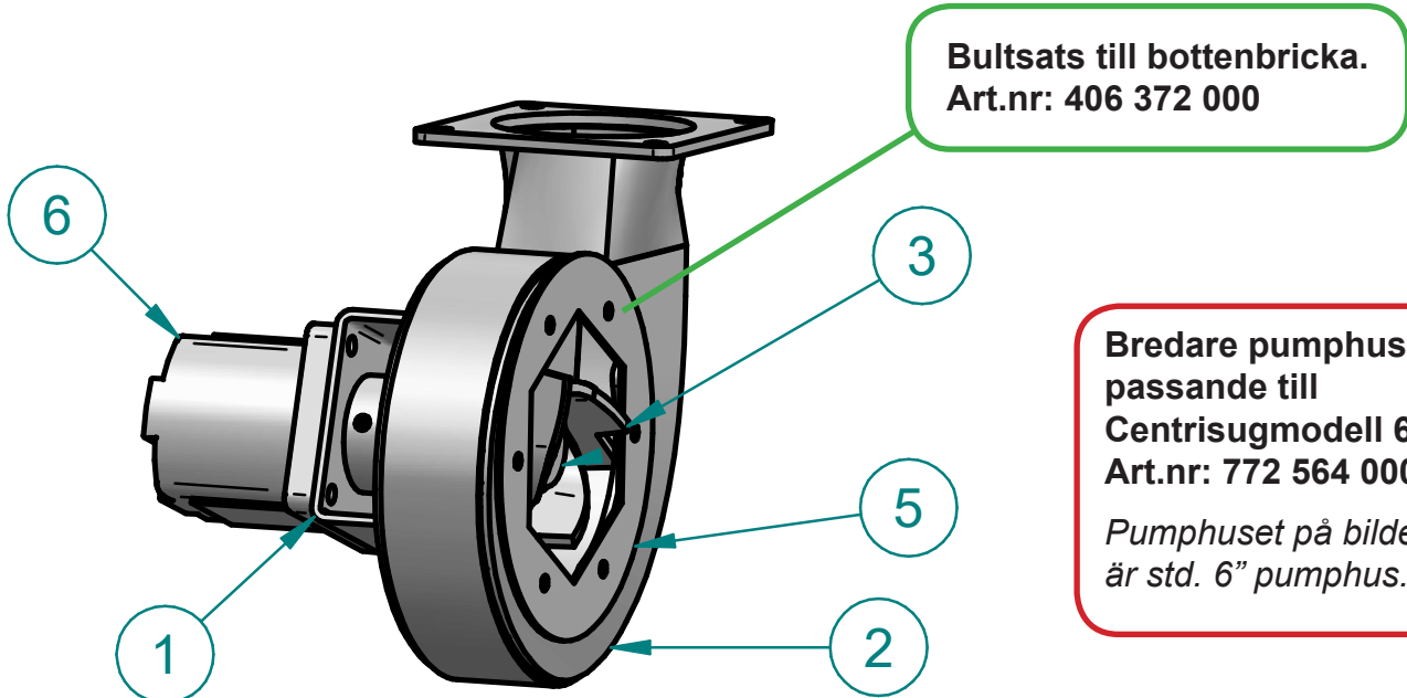
5" Art. nr: 764 785 000
